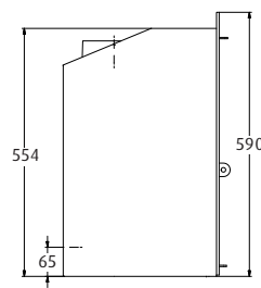
WESTFIRE.UNIQ.35 | INZET 3-ZIJDIG FRAM | GEWICHT: 75 KG
