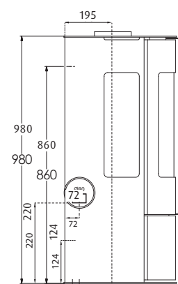
WESTFIRE.UNIQ.36 WESTFIRE.UNIQ.37 GEWICHT: 90 KG
