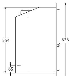
WESTFIRE.UNIQ.35 | INZET 4-ZIJDIG FRAM | GEWICHT: 75 KG
