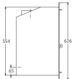
WESTFIRE.UNIQ.35 | INDSATS 4-SIDET RAMME VÆGT: 75 KG
