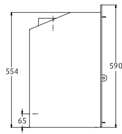
WESTFIRE.UNIQ.35 | INDSATS 3-SIDET RAMME VÆGT: 75 KG
