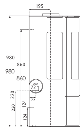
WESTFIRE.UNIQ.36 WESTFIRE.UNIQ.37 VÆGT: 90 KG
